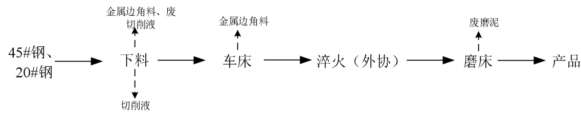
图 2-2 项目生产工艺流程图
